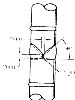
ث- جوش نیمه جناغی دوطرفه
