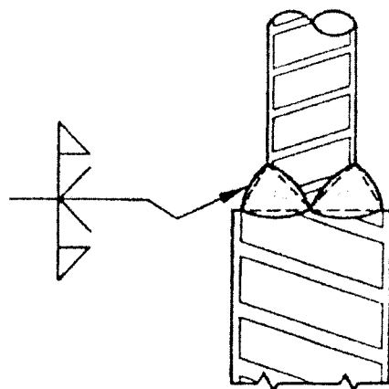
شکل ۸-۱۷ جزئیات اتصال نوک به نوک بدون پشت بند برای آرماتور با قطرهای متفاوت
