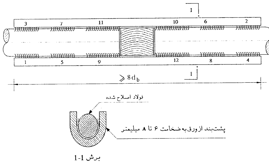
شکل ۸-۱۵ اتصال مضاعف
